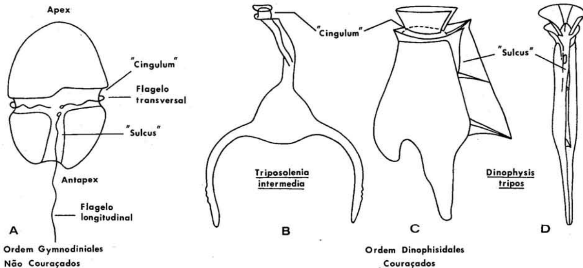
Figura 1 — Morfologia de dinoflagelados: A — Não couraçados. B-D — Couraçados. (Segundo EVITT, 1969 in CHÂTEAUNEUF e REYRE, 1974, p. 52)
