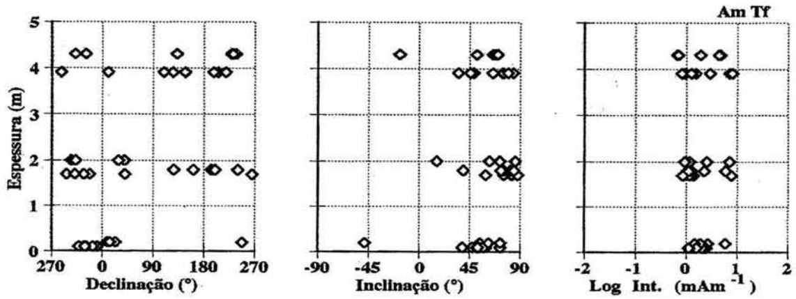
Fig. 2 – Representação dos valores de declinação, inclinação e intensidade relativos ao perfil de Salgueiro (1 - amostras Tf).
