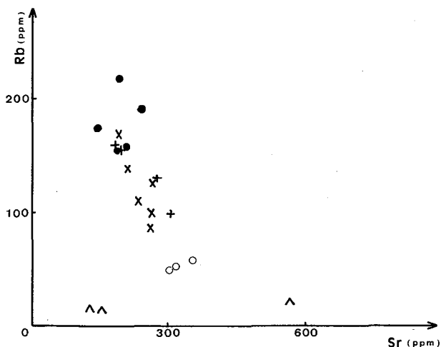
Fig. 9 — Diagrama Rb-Sr.
