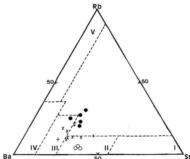
Fig. 11 — Diagrama ternário R-Ba-Sr de BOUSEILEY & SOKKARY (1975). I - dioritos; II- granodioritos e quartzodioritos; III - granitos anómalos; IV - granitos normais; V - granitos fortemente diferenciados.
