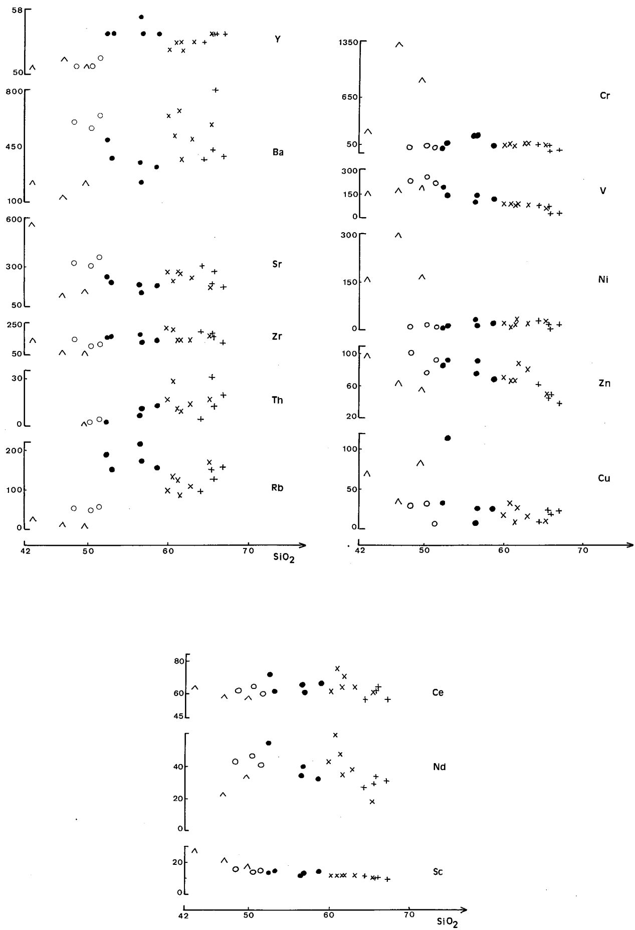
Fig. 7 — Diagramas de distribuição dos elementos menores (ppm) com SiO 2 (%).
