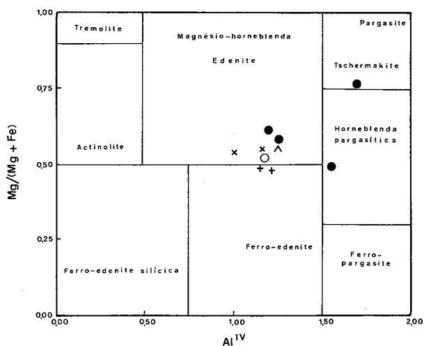
Fig. 13 — Variação química das anfíbulas cálcicas, expressa em função do número de átomos por fórmula unitária (Mg/Mg+Fe - Al IV ). Versão modificada da recomendada pela IMA para classificação das anfíbulas cálcicas.
